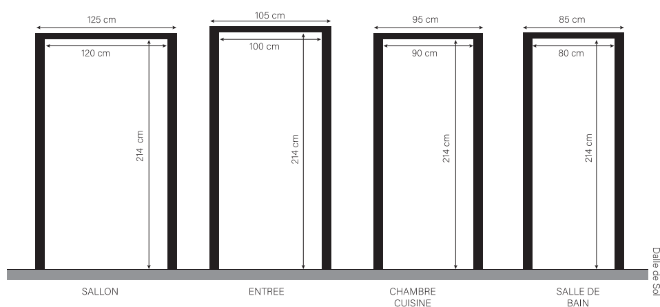
Dimension du pré-cadre (avec dalle de sol)
