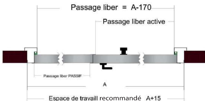
COUPE AA
