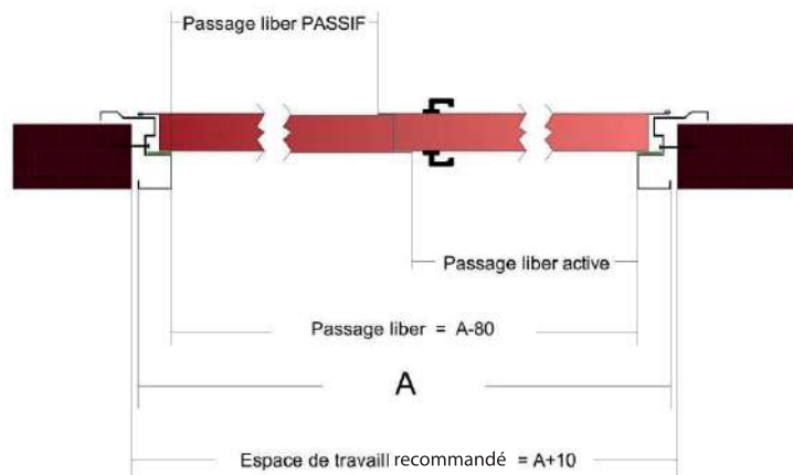
COUPE AA
