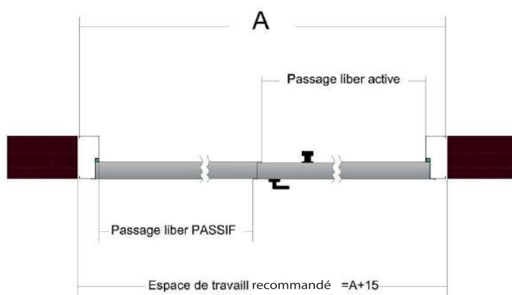
COUPE AA
