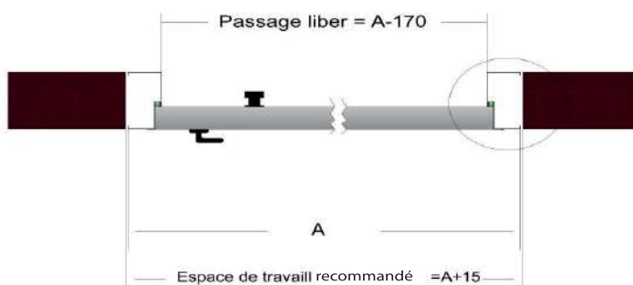
COUPE AA
